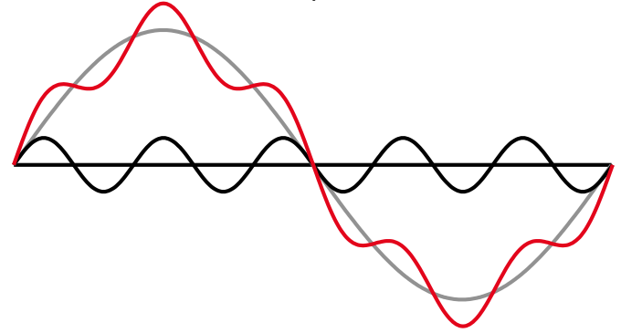
Courant total comme la somme de l'harmonique fondamentale et de la 5 ème harmonique
