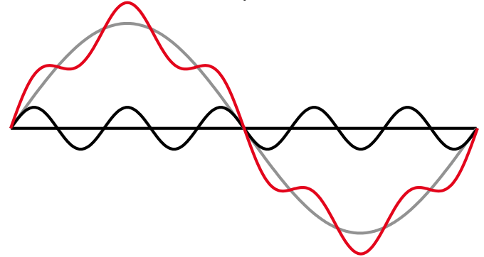
Courant total comme la somme de l'harmonique fondamentale et de la 5 ème harmonique
